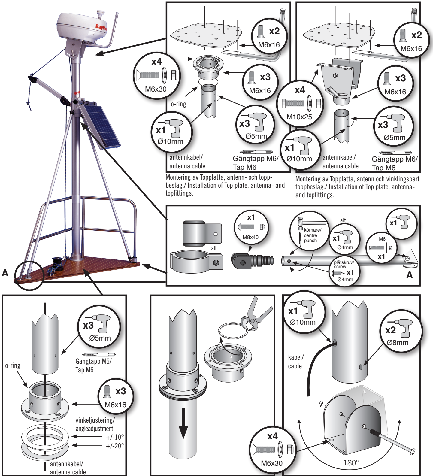
För genomgående däcksfäste måste en metallring plockas bort./ For mounting through the deck, a metalring has to be removed.
